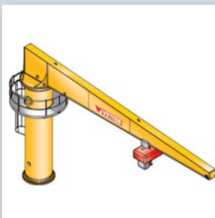
Schwenkkrane mit Wartungsbühne Slewing jib crane with maintenance platform
