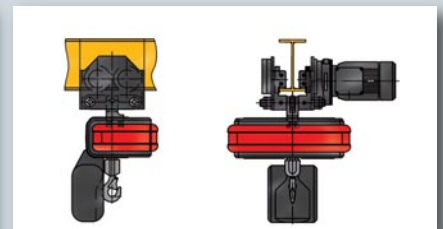
ELECTROLIFT® SiCC mit Elektrofahrwerk ELECTROLIFT® SiCC with electric trolley
